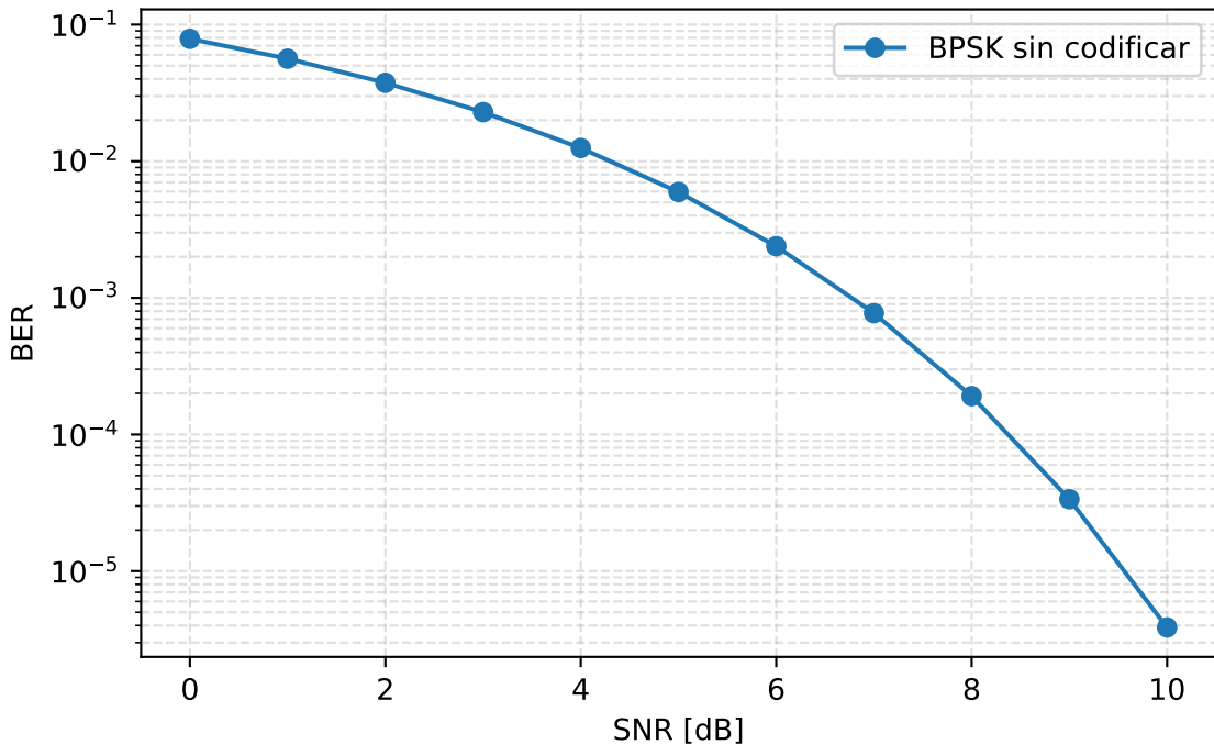
Curvas BER vs SNR
